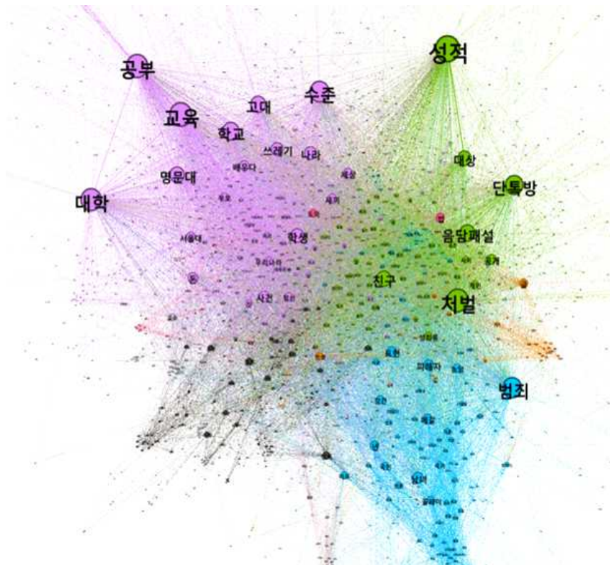
그림 1. 단어동시출현 네트워크
